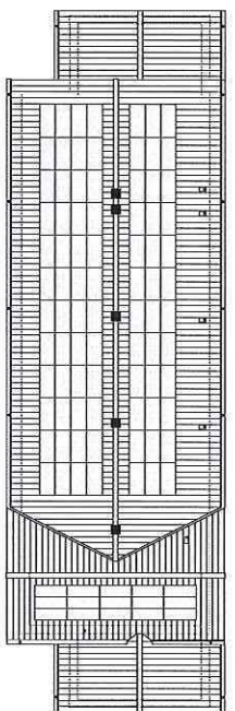
dakvlak blok B, D
